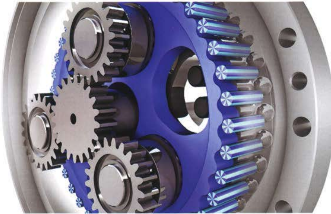
Die für Zykloidgetriebe typische Kraftübertragung über Bolzen und Rollen sorgt für einen hohen Wirkungsgrad und geringen Verschleiß Foto: Nabtesco
